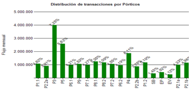
Gráfico 3: Distribución de transacciones del mes por pórtico de cobro. Fuente: Reporte SICE N° 29 de fecha 16.06.2016.
